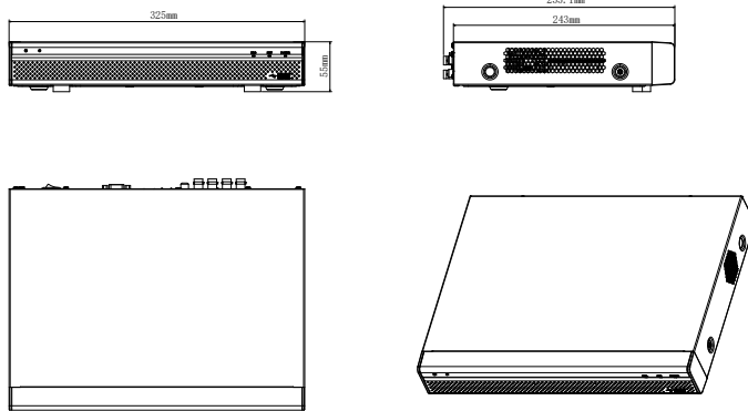
DHI-XVR5116H-4KL
